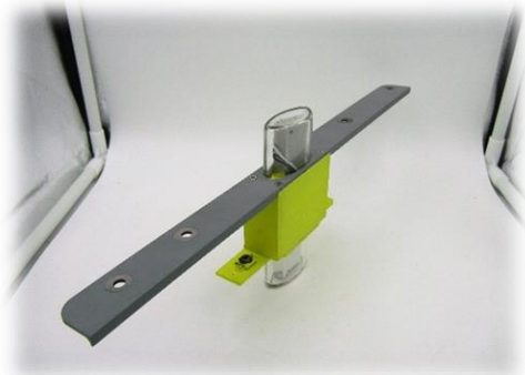
翼尖燈 Wingtip
